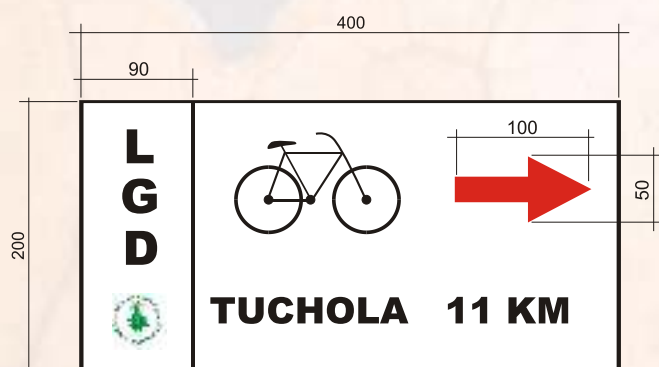
TABLICA INFORMACYJNA-DROGOWSKAZ
